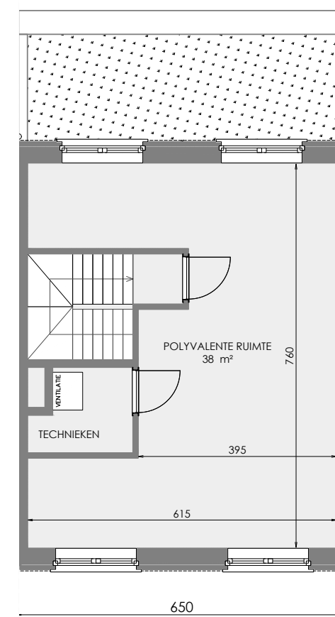
VERDIEPING 2
