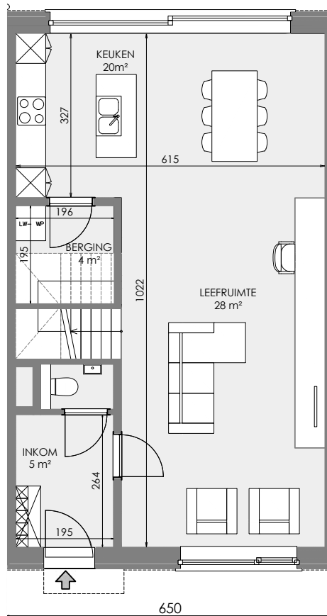
GELIJKVLOERS
