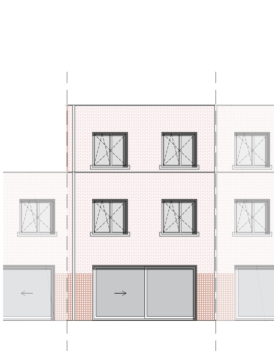
NOORDGEVEL
