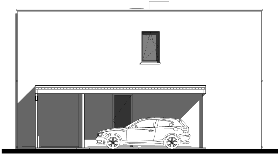
zijgevel links
