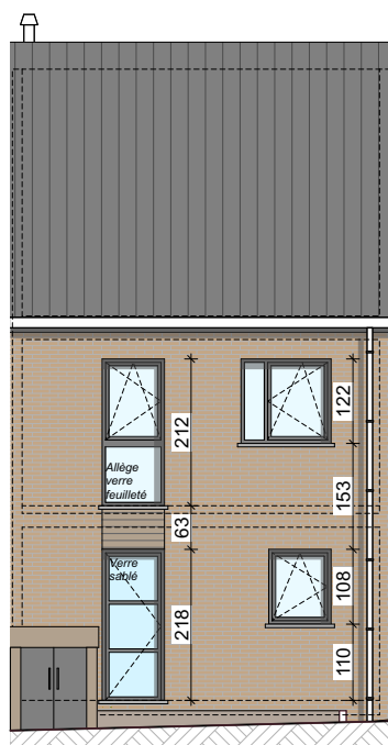
Façade avant
