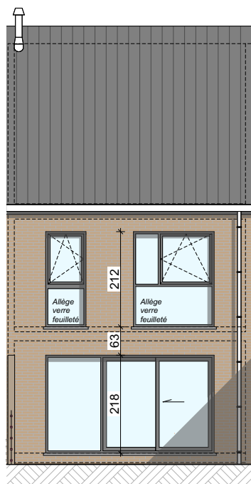
Façade arrière
