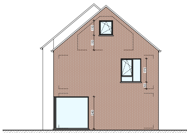
Façade latérale gauche
