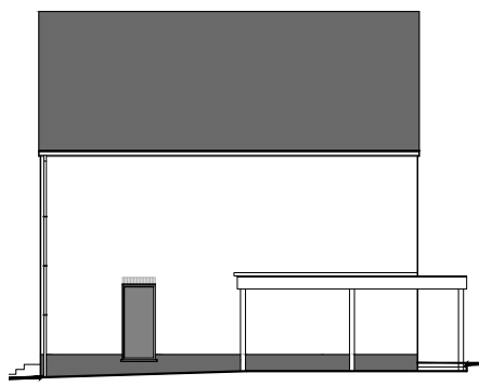
Zijgevel rechts
