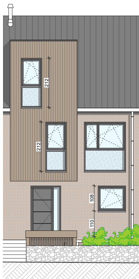
Façade avant
