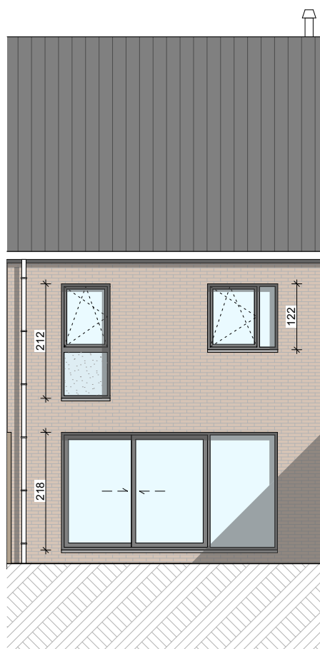
Façade arrière
