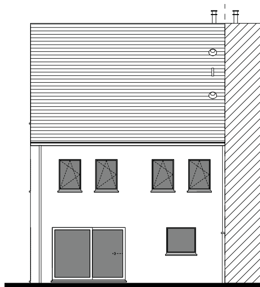
Achtergevel
